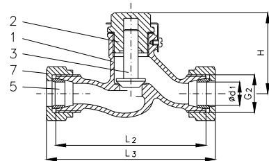
Art.Nr. 21.75.05 Lötkegelverschraubung
